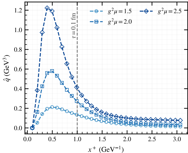
(a) Jet quenching parameter
